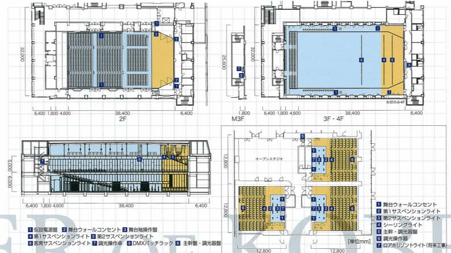
平断面図 [単位mm]
